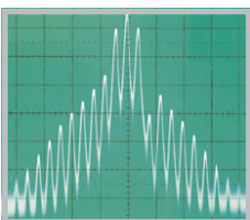
Señal de AF modulada en AM
