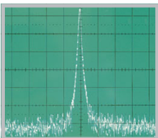
Señal de AF sin modular
