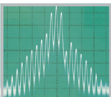
Signal HF modulé en Amplitude
